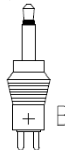
Klinkenstecker/ jackplug ø3,5x15mm
